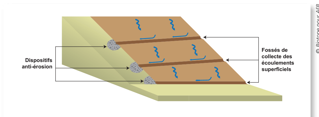
Figure 31. Collecte puis dérivation des écoulements superficiels issus du chantier à l'aide de fossés en série aboutissant à des dispositifs anti-érosion (fiches Lutter n°7 et n°8). Les eaux ainsi concentrées sont soit infiltrées soit transportées vers un dispositif de traitement des sédiments.
