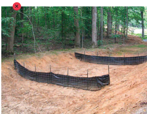
Les barrières perméables en géotextile ne sont pas tendues jusqu'aux talus du bassin de décantation.
