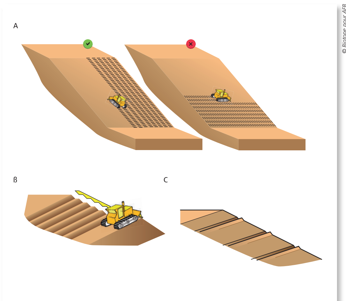
Figure 21. Exemples de microreliefs créés perpendiculairement à la pente : (A) empreintes par chenillage des sols ; (B) marches ; (C) sillons. Source : McCullah (2007).
