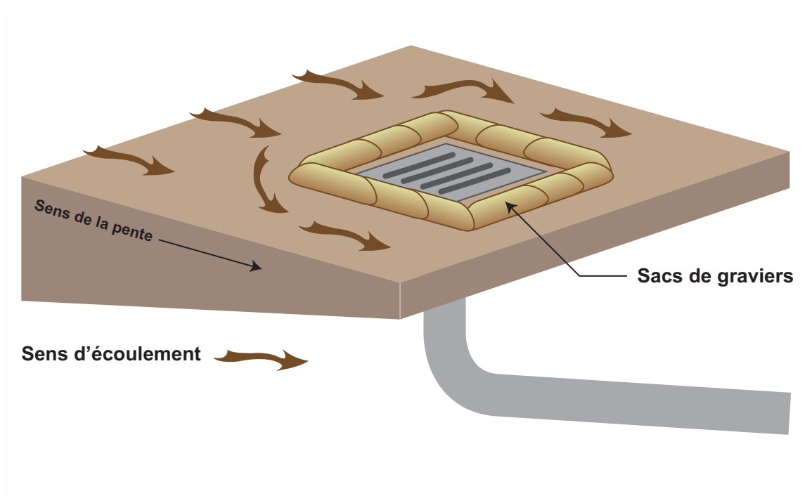
Figure 47. Exemple d'une protection de bouche d'égout : barrière périphérique en sac de graviers.
