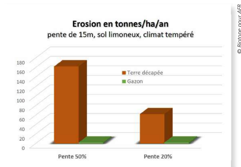
Figure 7. Taux moyen d'érosion des sols selon la pente et la nature des surfaces concernées. Tests réalisés sur des surfaces pentues de 15 m de long, des sols limoneux et sous un climat tempéré. Source : McCaleb et al. (2008).
